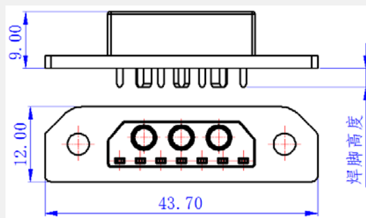
焊脚高度
